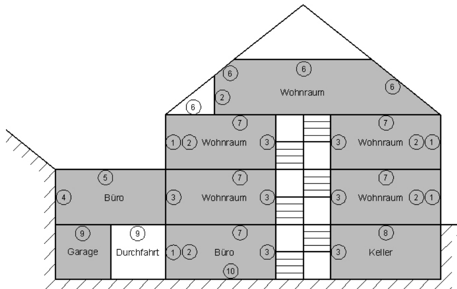
Abb. 4.8: Bauteilpositionen
