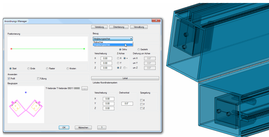
Abb. 1.3: Verbinder bei Riegelpaar mit variablem Winkel
