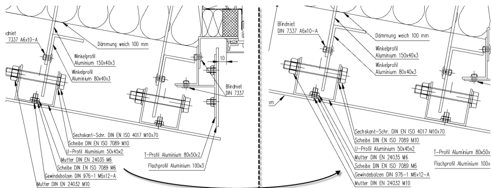
Abb. 5.12: Beschriftungen ordnen
