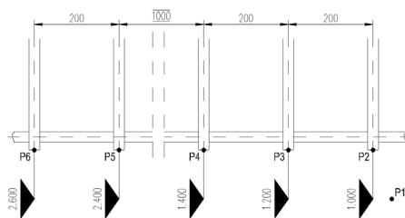
Abb. 5.8: Horizontale Höhenkoten
