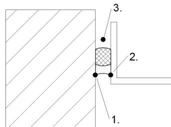
Abb. 1.13: Versiegelung Punktmodus
