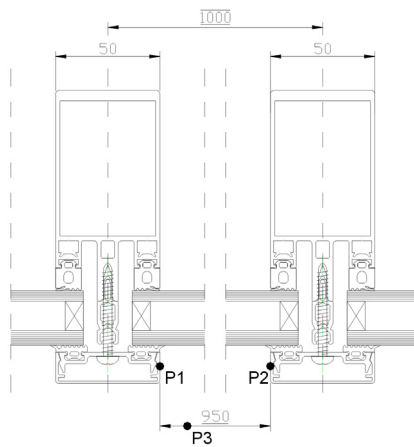
Abb. 4.7: Abgerissene Bemaßung
