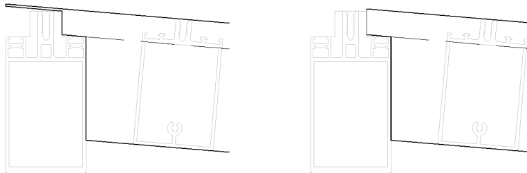
Abb. 1.1: Zuschnittsmodi: links Basis, rechts Fassade
