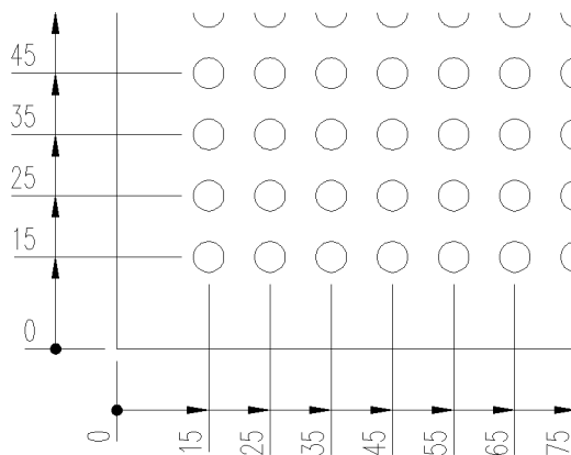
Abb. 4.3: Koordinatenbemaßung eines Lochblechs
