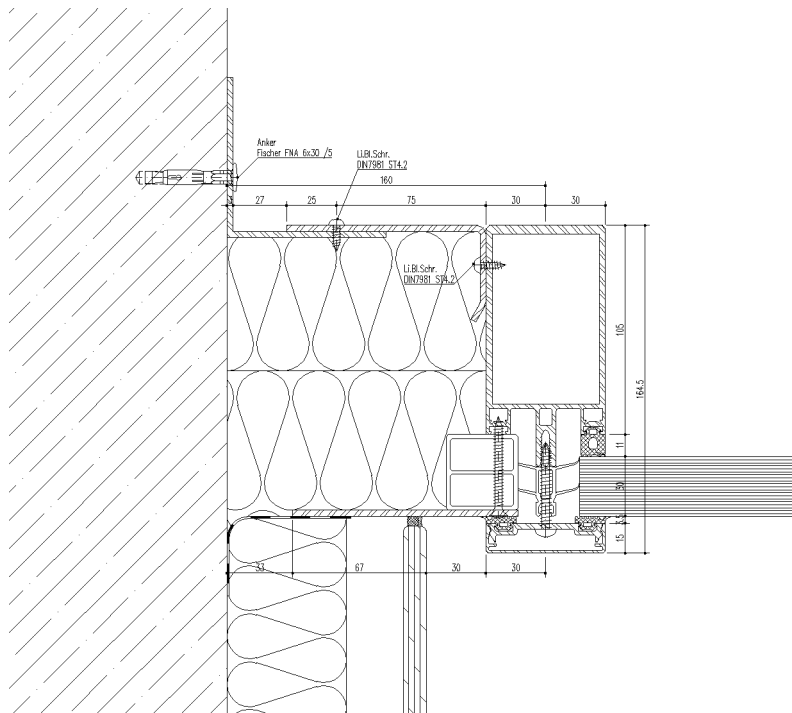
Abb. 3.4: Wandanschluß
