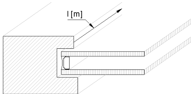
Abb. 3.9: Länge der Einspannung (Psi-Wert)
