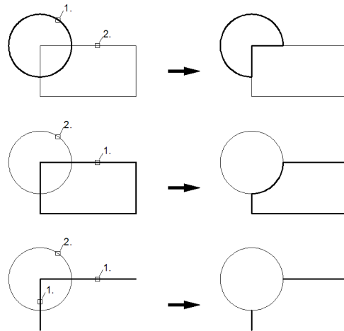
Abb. 5.6: Beispiele für gestanzte (geklinkte) Konturen
