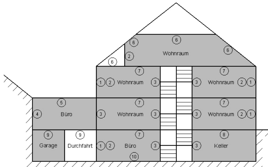
Abb. 3.8: Bauteilpositionen
