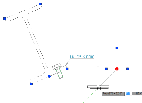
Abb. 1.1: Runder Griff zum Schieben von Objekten
