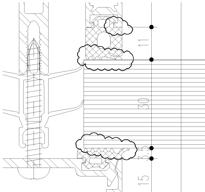
Abb. 3.5: Detail EPDM-Dichtung an Glasfüllung, geschlossene Hohlräume
