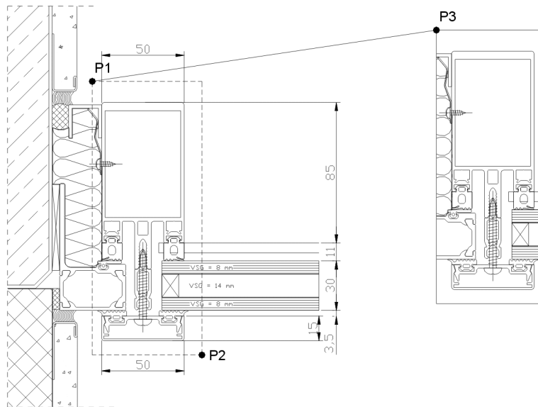
Abb. 5.2: Detail kopieren
