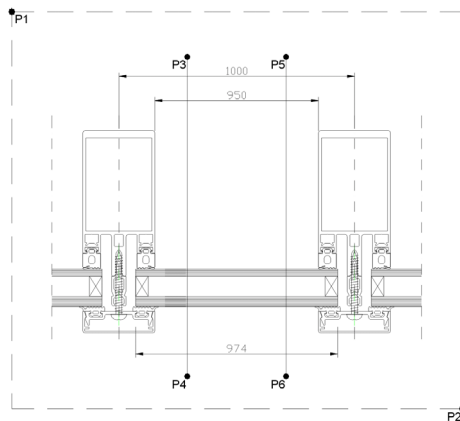
Abb. 4.5: Abriss
