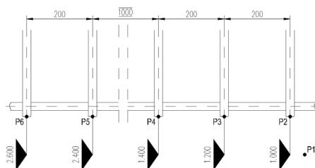
Abb. 4.8: Horizontale Höhenkoten
