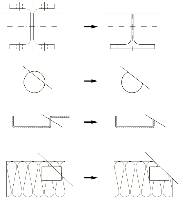
Abb. 5.5: Beispiele für Objekte kappen
