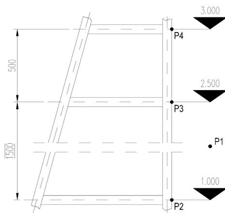
Abb. 4.9: Vertikale Höhenkoten
