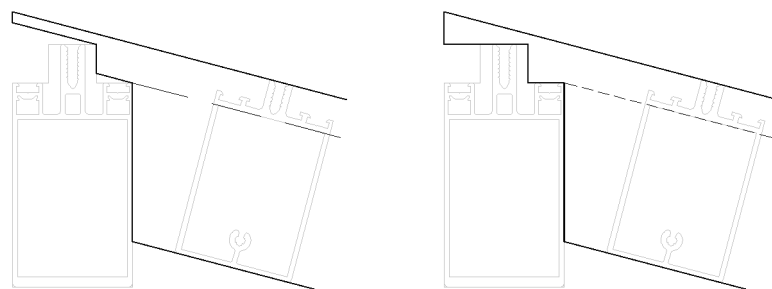
Abb. 1.2: Winkelschatten: links an, rechts aus
