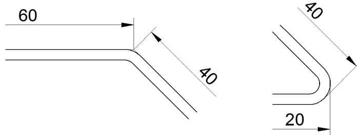
Abb. 1.5: Maßpunkte: links stumpfer Winkel, rechts spitzer Winkel
