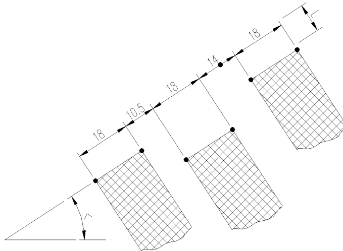
Abb. 4.1: Kettenbemaßung
