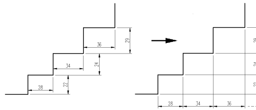
Abb. 4.10: Bemaßung ordnen
