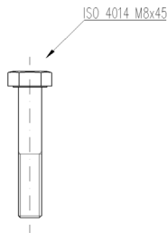
Abb. 4.4: Beschriften einer Schraube
