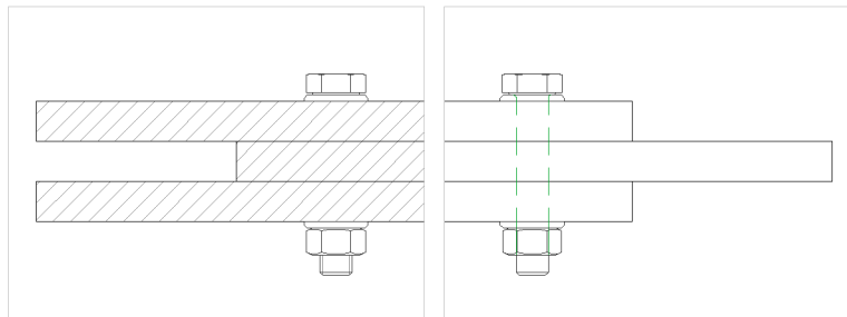
Abb. 5.8: Verdeckungsmodi: links Aus, rechts Ein
