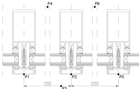
Abb. 4.6: Abgerissene Definitionsmaße
