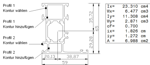
Abb. 3.1: Schwerpunkt und Momente von Profilen
