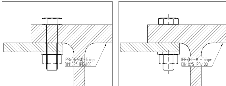
Abb. 5.7: Verschraubung sichtbar und verdeckt
