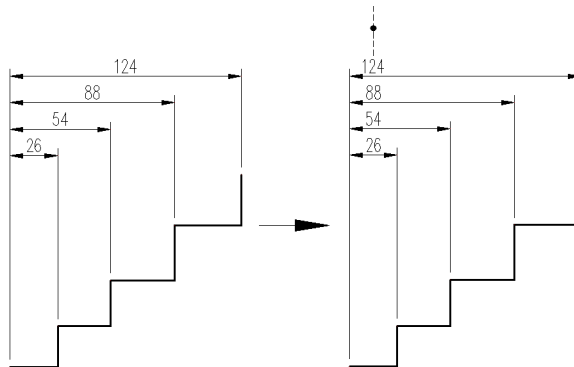
Abb. 4.11: Maßtexte ordnen
